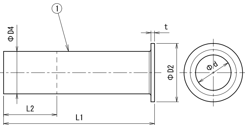
BMH-22, 28, 150, 200 塩ビ管加工品（ロックナット無し）
